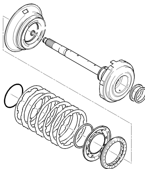
F E1 Clutch
