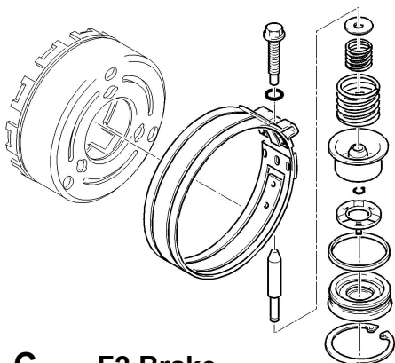
C F2 Brake
