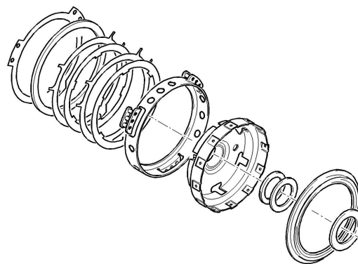
D F1 Brake
