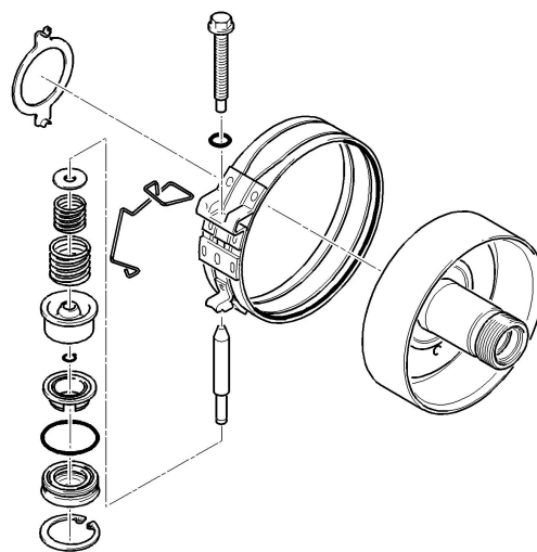
B F3 Brake
