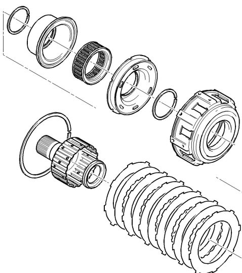
E E2 Clutch
